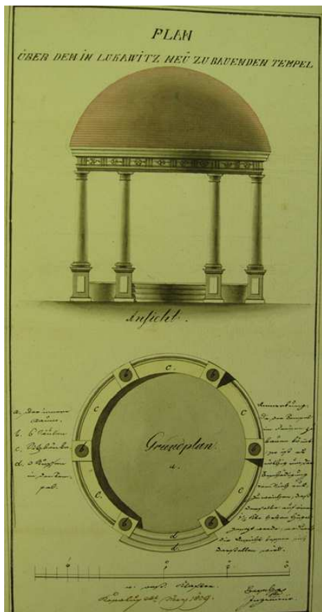
Obr. č. 5 Plán letohrádku z roku 1809
