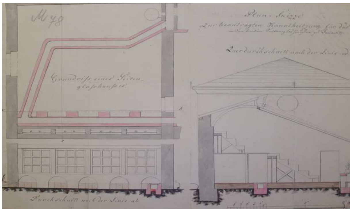
Obr. č. 6 Plán vytápění skleníku z roku 1850
